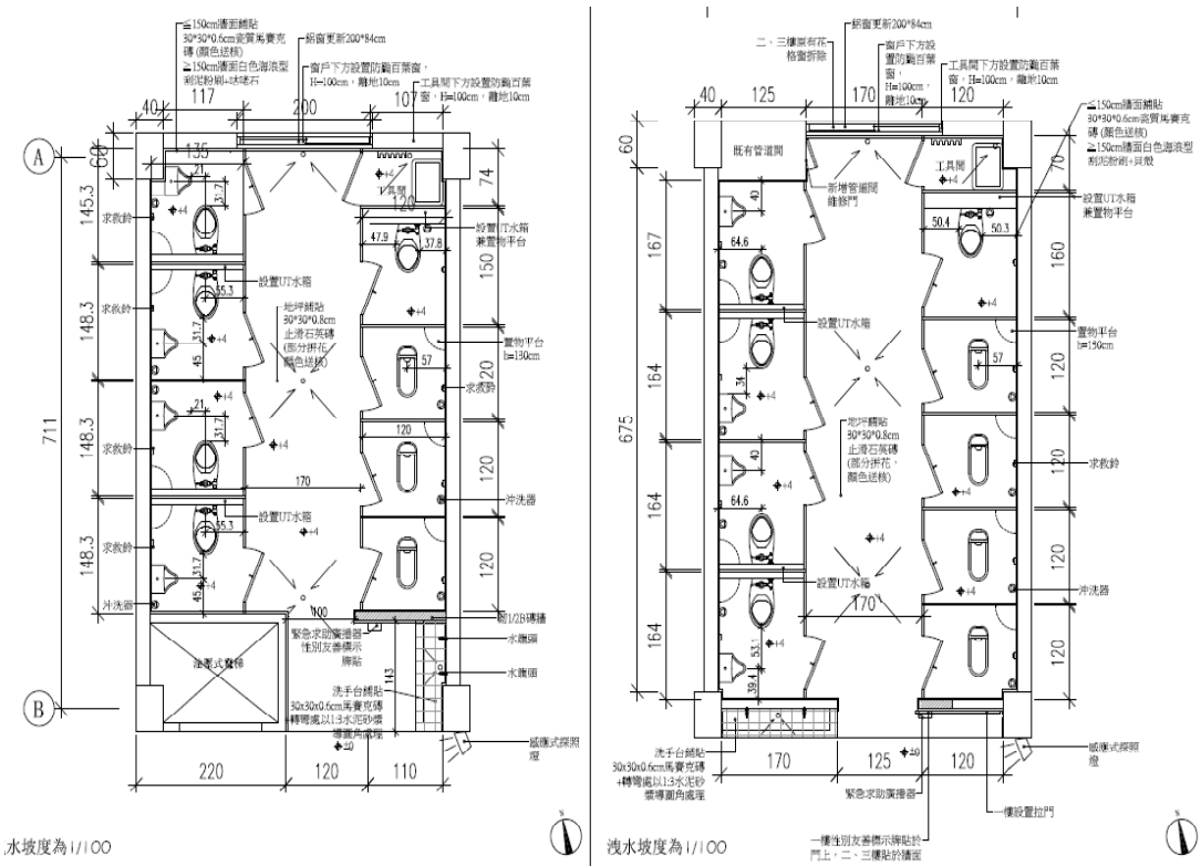
1.壹層左側廁所整修後平面圖
